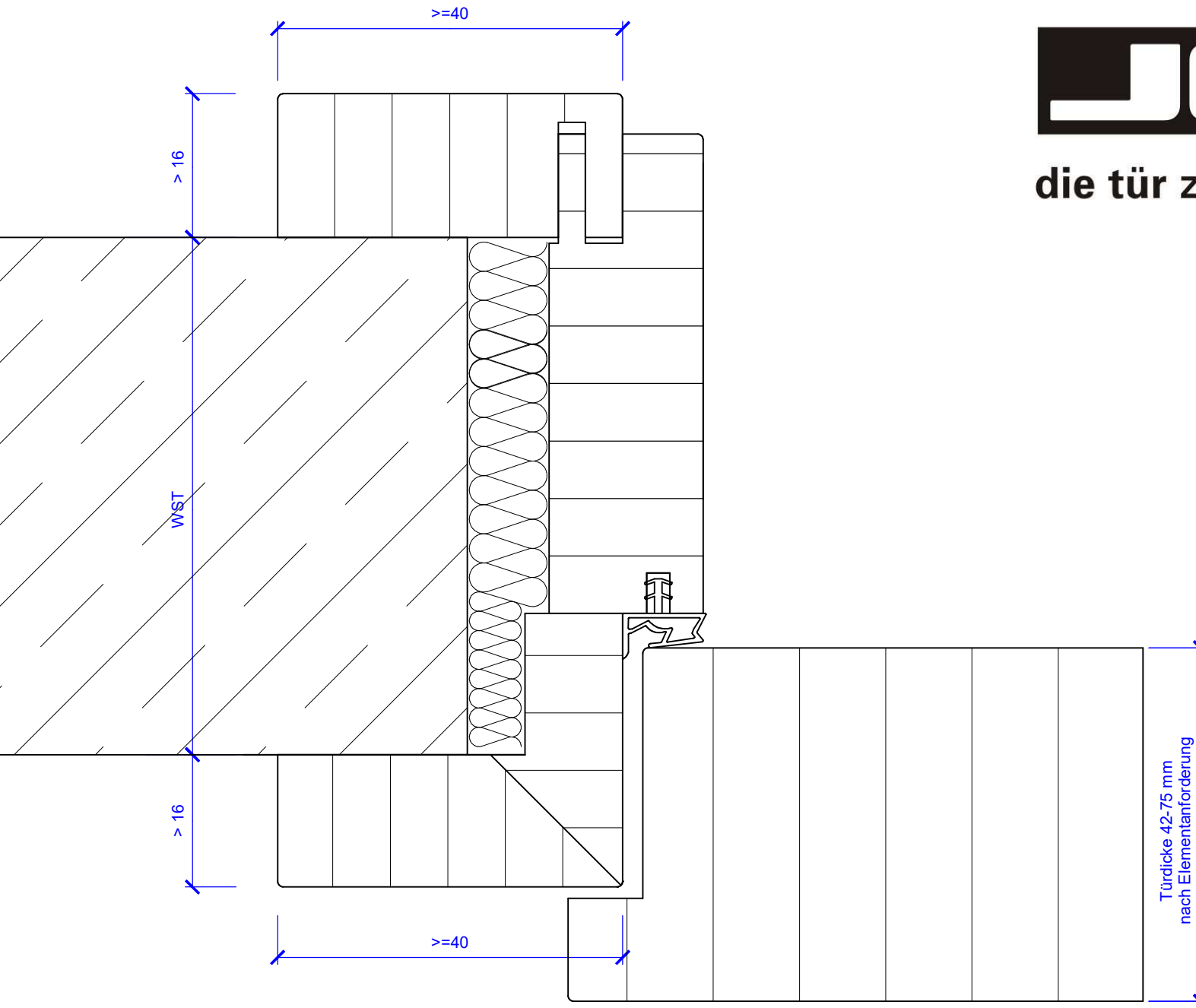
Holzumfassungszarge mit zwei Dichtungsebenen, Dichtungsebene lose, Türblatt gefälzt
